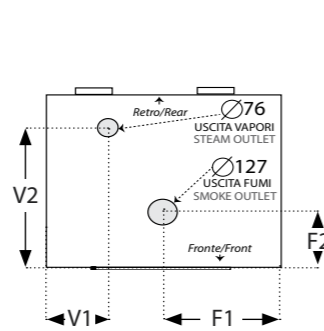
Vista dall'alto - View from the top
